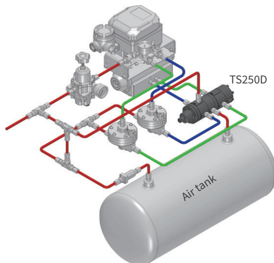
Double actuator
